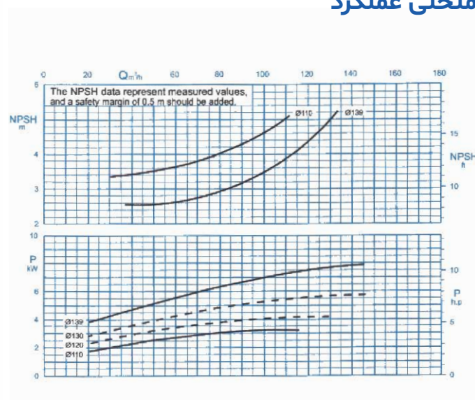
منحنی عملکرد
