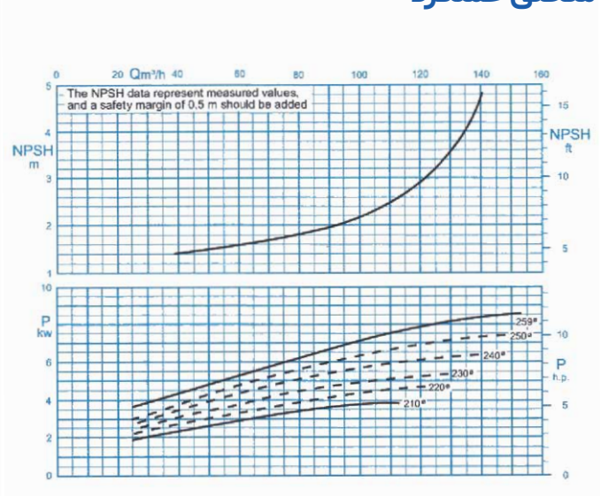
منحنی عملکرد
