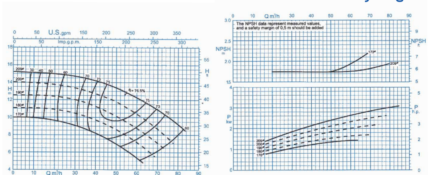
منحنی عملکرد
