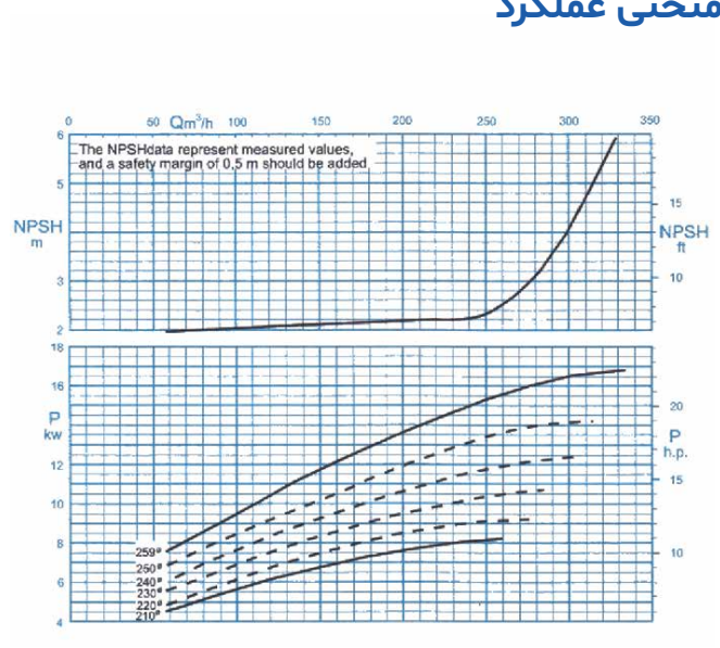
منحنی عملکرد
