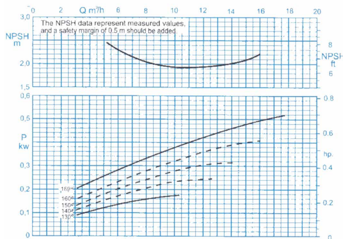
منحنی عملکرد
