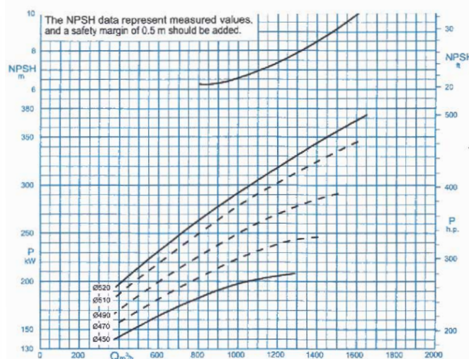
منحنی عملکرد
